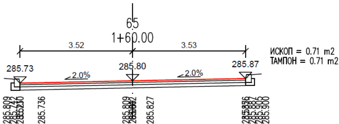
Слика 2 Пресек на локалната улица „Филип 2“ во Свети Николе
